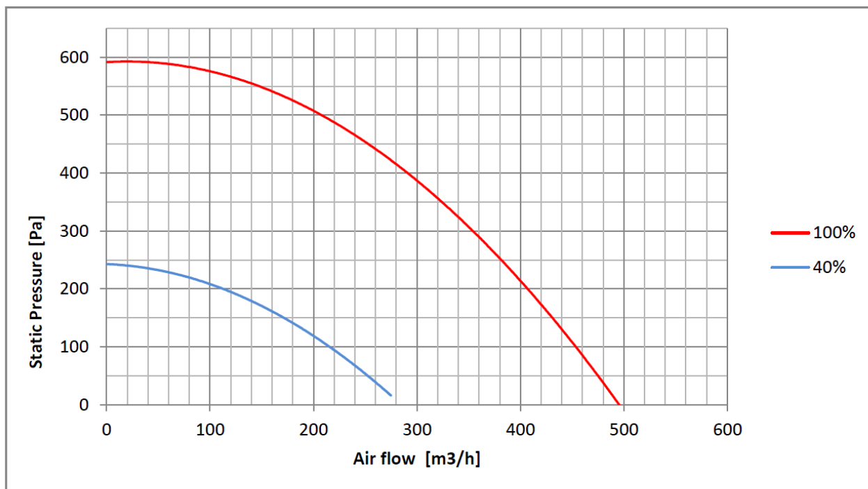
Rys.2 - Wykresy wydajności centrali OnyX Dream 400
