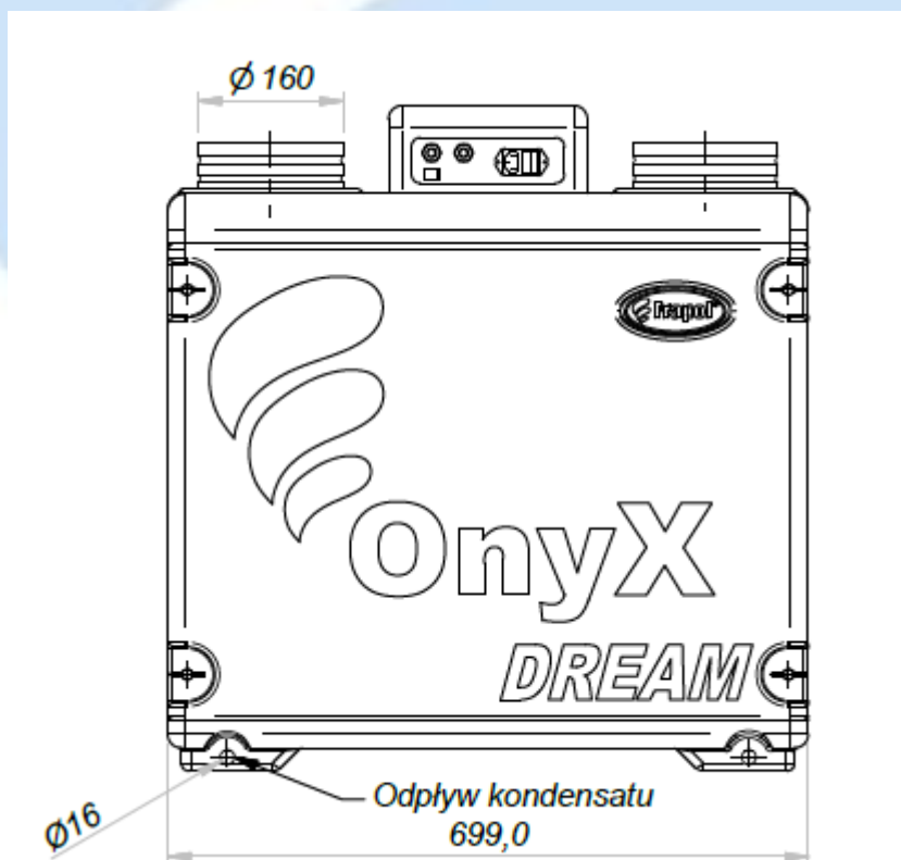
Rys.4 - Układ odprowadzania kondensatu z centrali OnyX Dream
