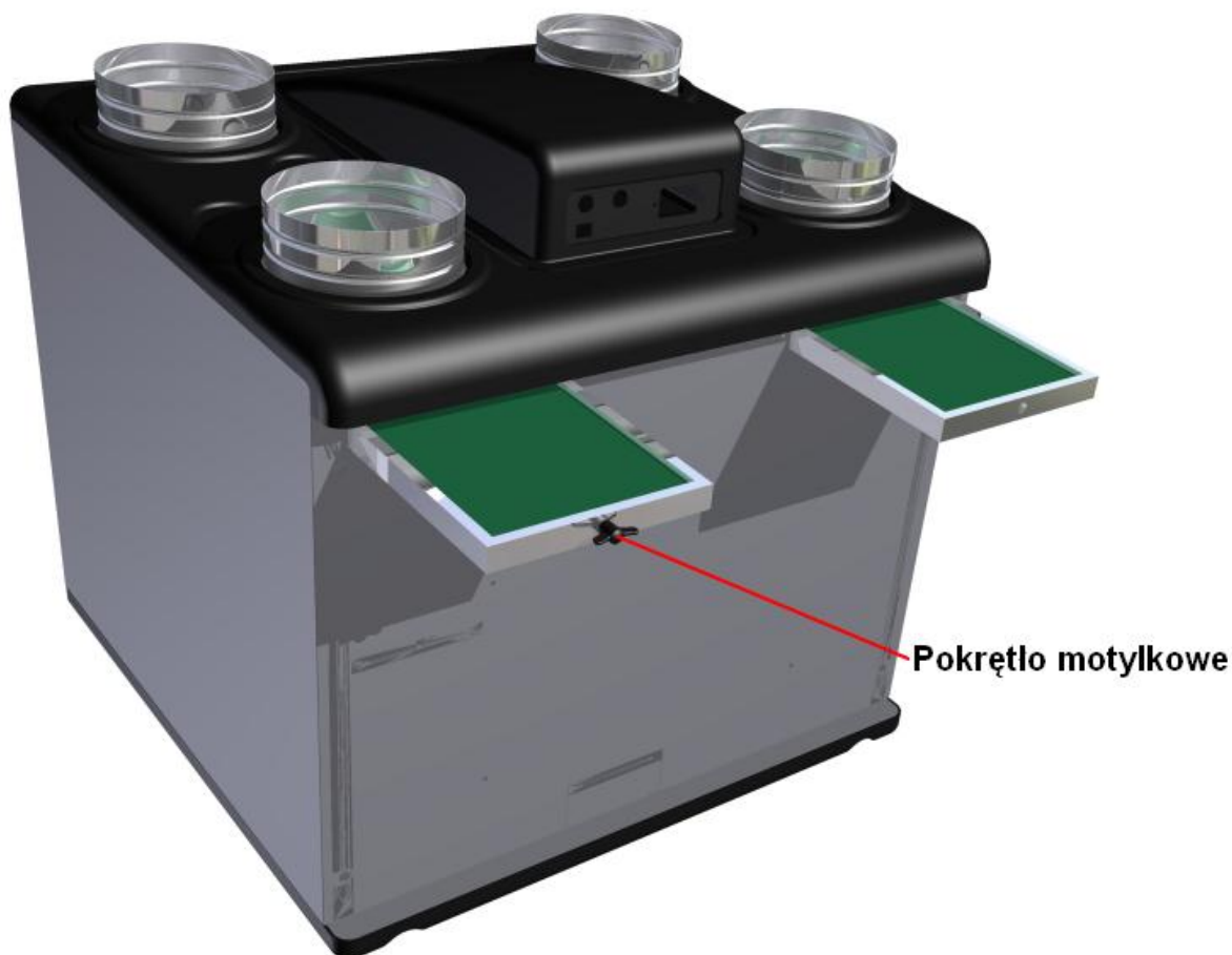
Rys.7 - Wymiana filtrów centrali wentylacyjnej OnyX Dream 400
