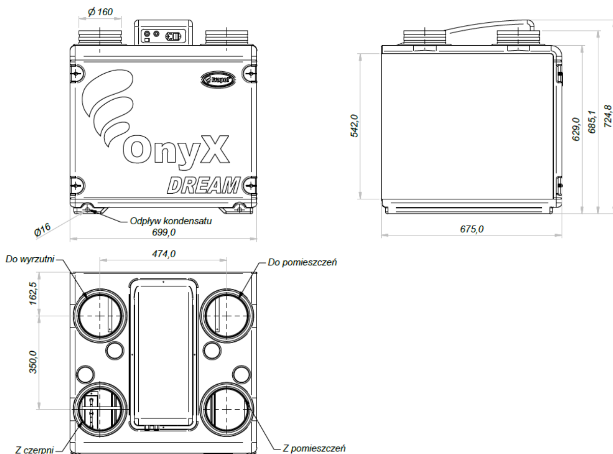
Rys.1 - Wymiary zewnętrzne centrali wentylacyjnej OnyX Dream 400
