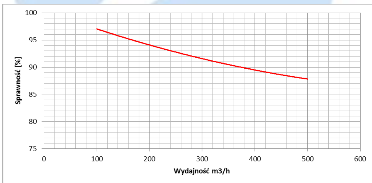
Rys.3 - Krzywa sprawności centrali OnyX Dream 400
