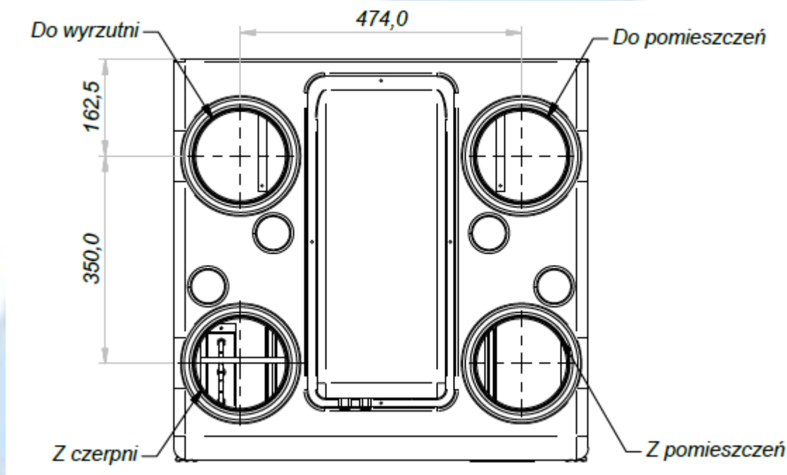
Rys.5 - Rozmieszczenie przyłączy wentylacyjnych w centrali OnyX Dream
